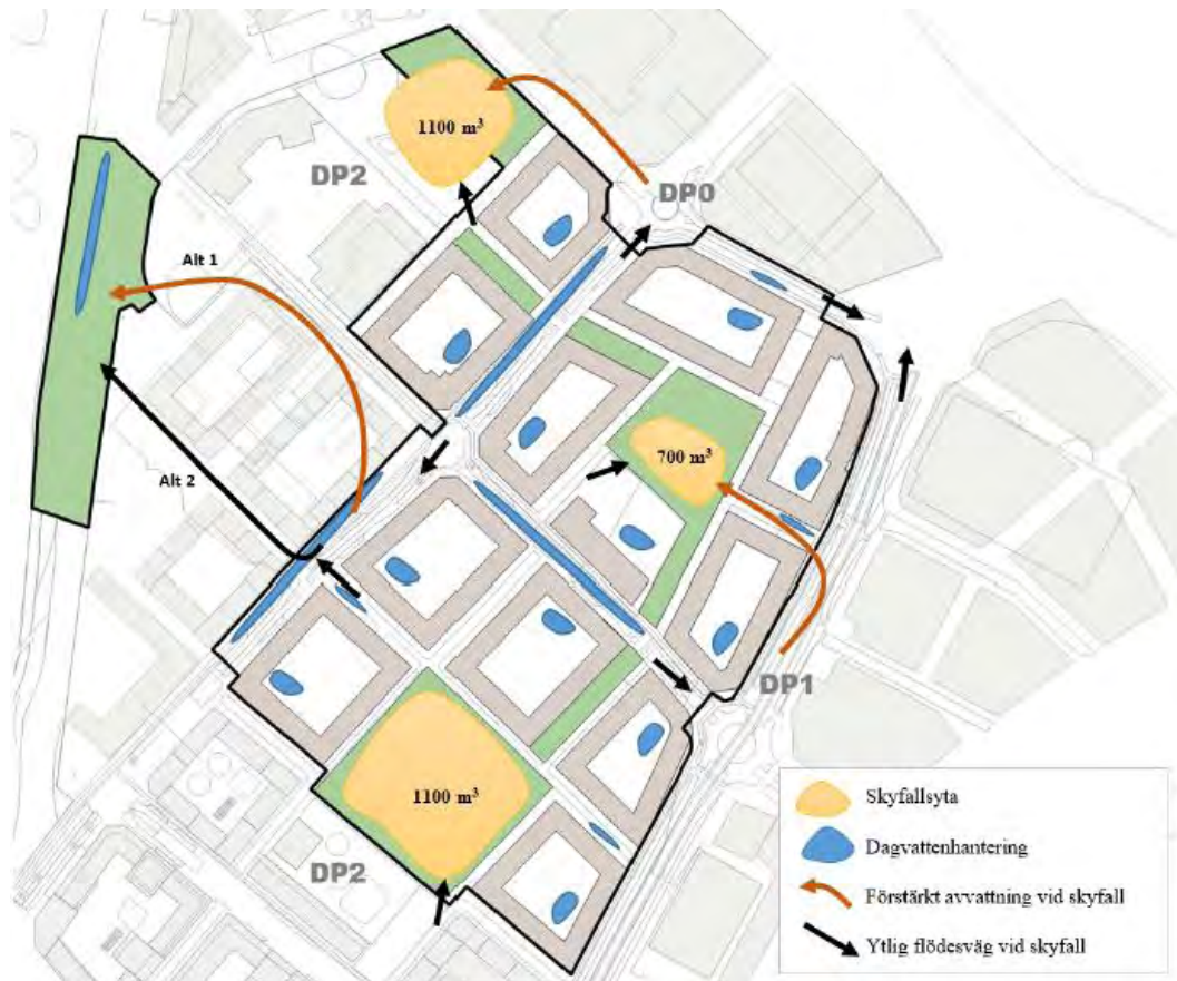
Figur 44. Principskiss över dagvatten- och skyfallshantering inom DP3. Placering och storlek på anläggningarna är endast ungefärligt redovisade (KoV 2022-05-31)
