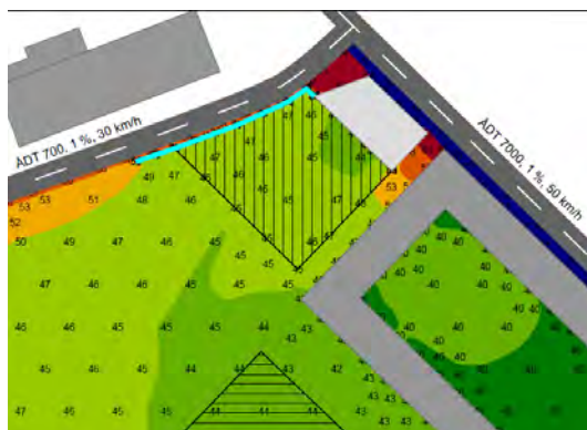
Ekvivalenta bullernivåer på förskolegård med 2 m hög bullerskärm.
